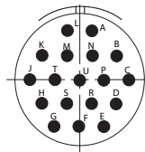
15-18/14-18 D18, 18 # 20, I
