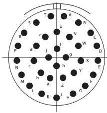
19-32/18-32 F32, 32 # 20, I
